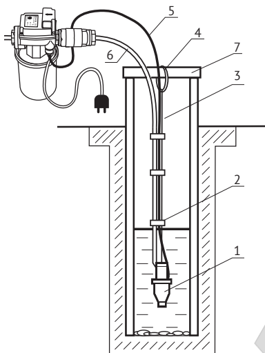
Рис.2 Схема установки
