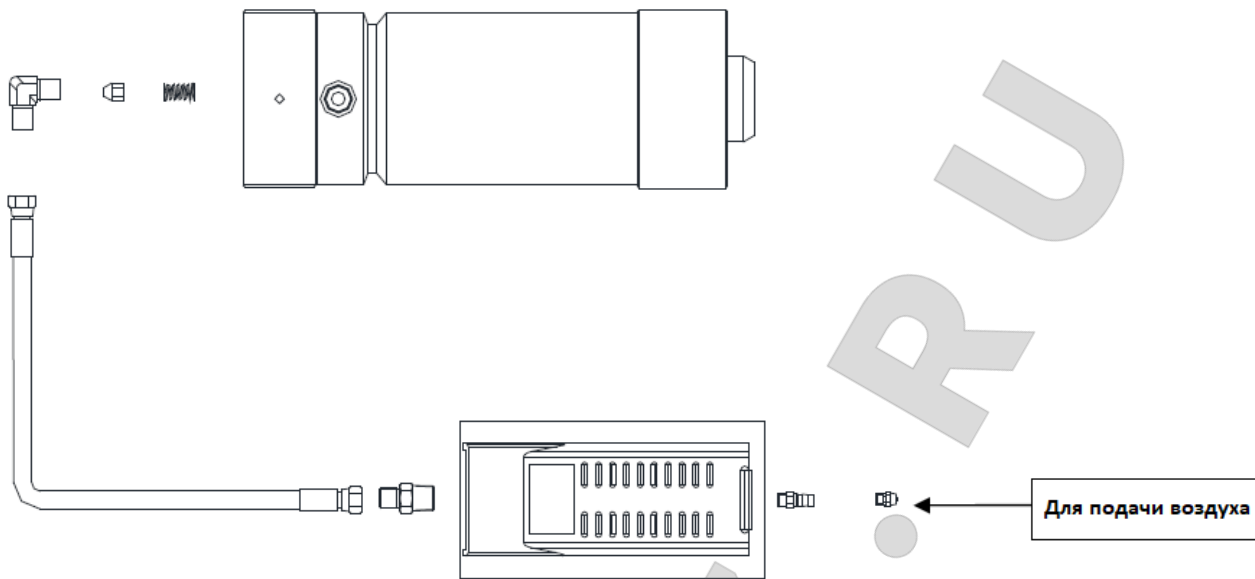
Рисунок 4. Подключение линии
