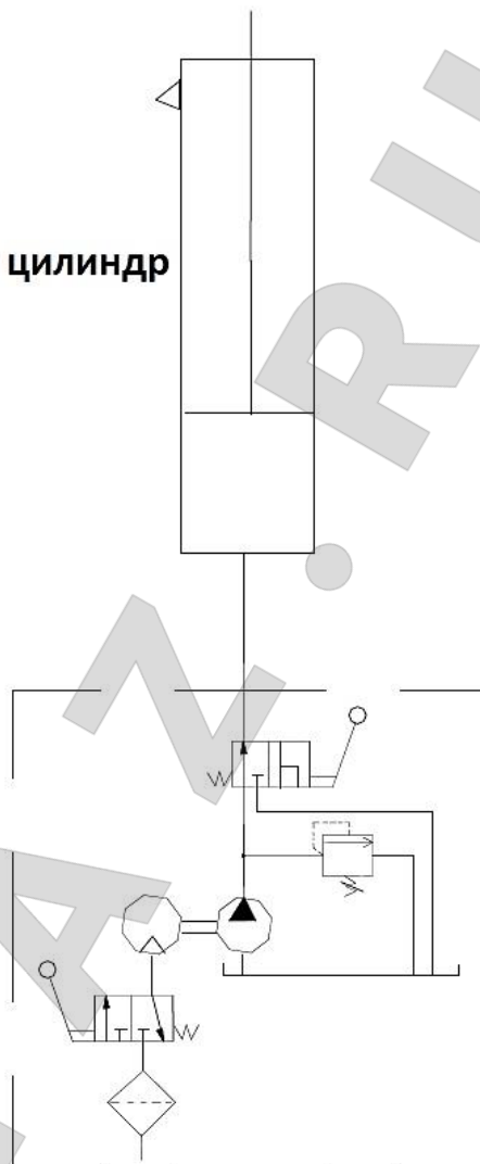
Рисунок 3. Гидравлическая схема
