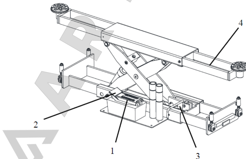
Рисунок 5. Устройство управления траверсой
