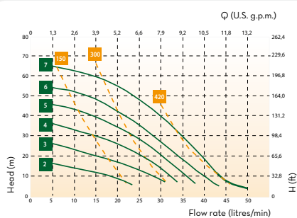
PIUSI MA 130
