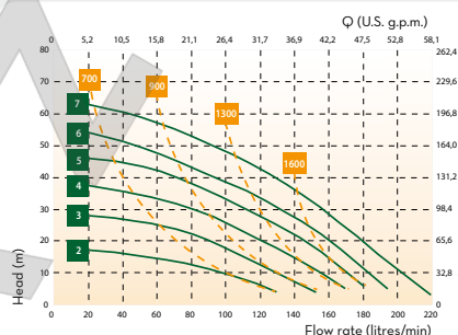
PIUSI MA 190
