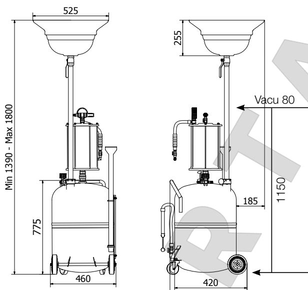
Vacu-DRAINER 80 / Easy-DRAINER 80
