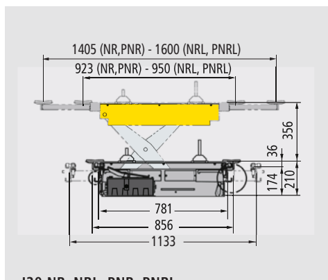
J20 NR J20 NRL J20 PNR J20 PNRL
