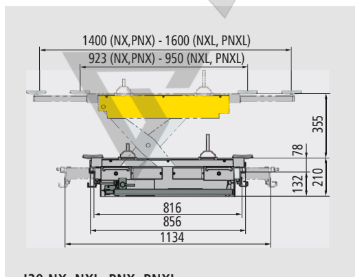
J20 NX J20 NR J20 PNХ J20 PNXL
