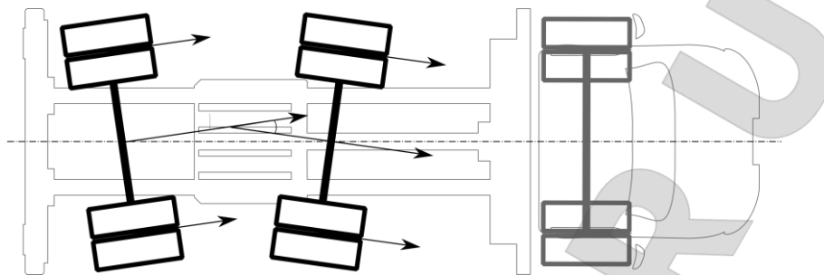
Рисунок Д.8 – Угол расхождения тандема (Scrub angle)
