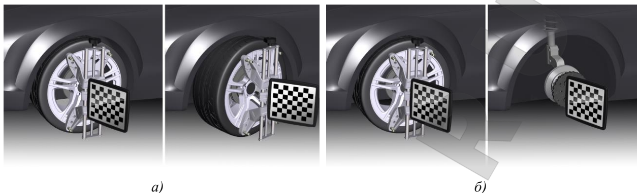
Рисунок 3.46 – Установка колеса в режимах а) в повороте; б) при снятом колесе
