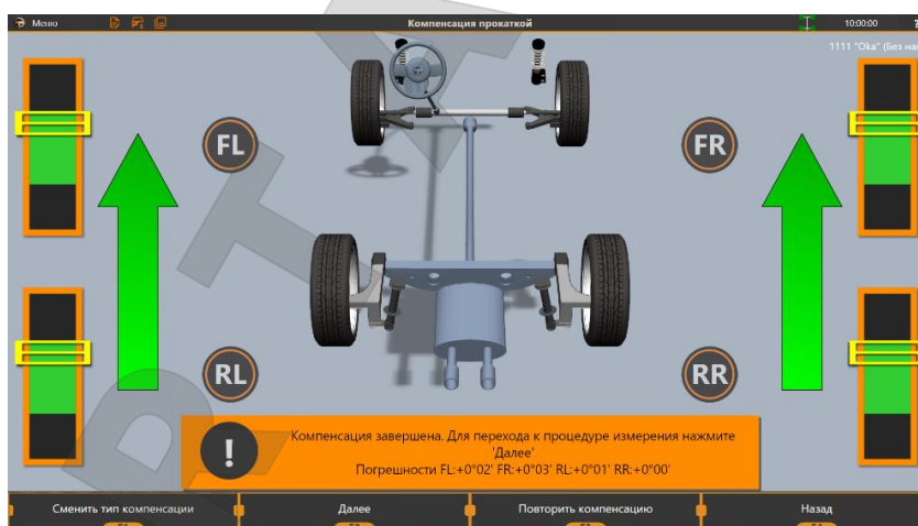
Рисунок 3.29 – Результат компенсации прокаткой
