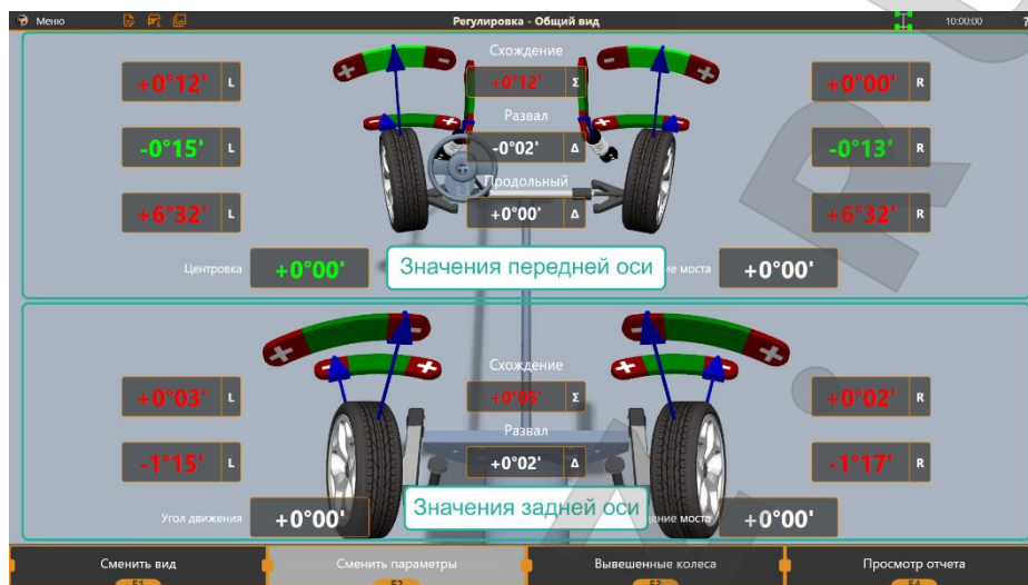
Рисунок 3.38 – Пример экрана в режиме регулировки
