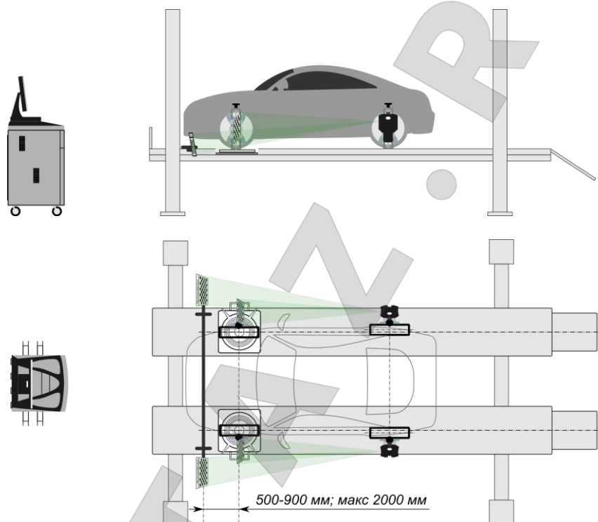
Рисунок Б.1 – Пример размещения прибора и автомобиля на рабочем месте
