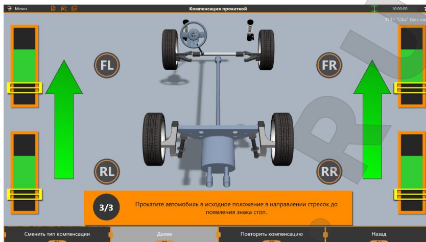
Рисунок 3.28 – Прокатка автомобиля вперёд
