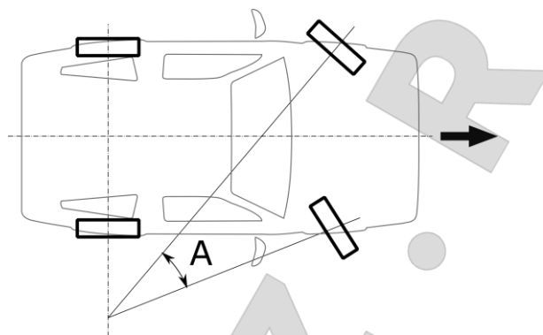
Рисунок Д.2 – Обратное схождение в повороте
