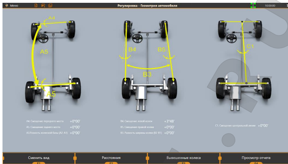
Рисунок 3.42 – Пример экрана в режиме регулировки геометрии подвески
