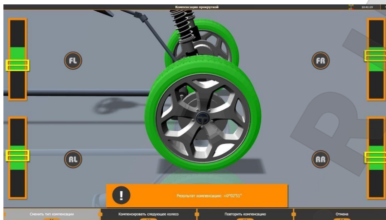
Рисунок 3.24 – Пример результатов компенсации
