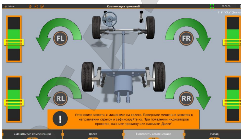
Рисунок 3.25 – Установка мишеней для компенсации методом прокатки
