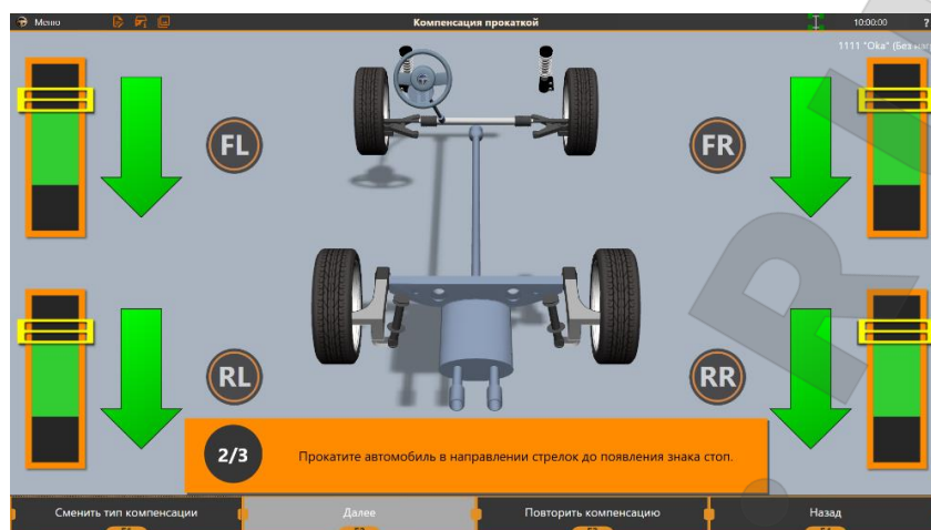
Рисунок 3.26 – Прокатка автомобиля назад
