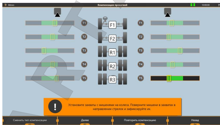
Рисунок 3.31 – Установка мишеней для компенсации прокаткой
