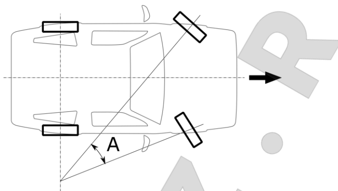
Рисунок Ж.2 – Обратное схождение в повороте
