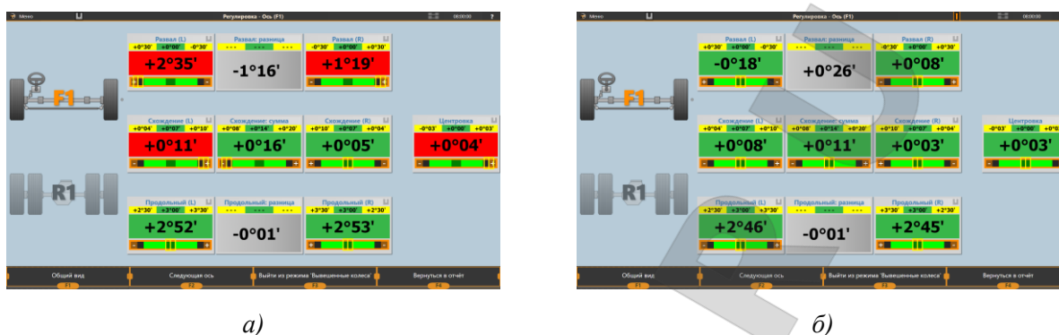
Рисунок 3.48 – Значения углов установки для вывешенного колеса
