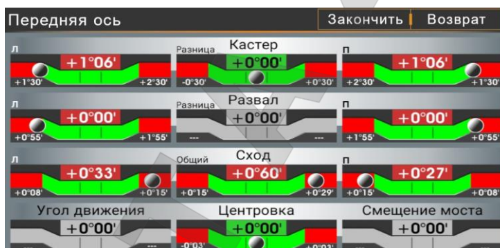
Рисунок 3.64 – Просмотр параметров регулировки в мобильном приложении
