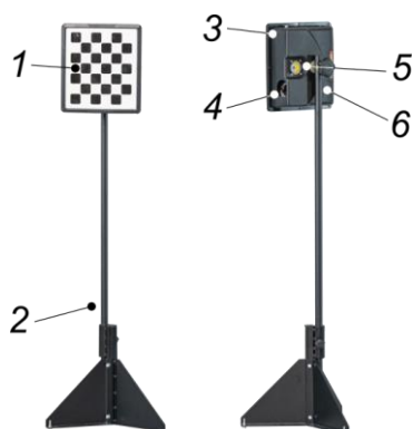
Рисунок Г.1 – Состав измерительного лазерного щупа
