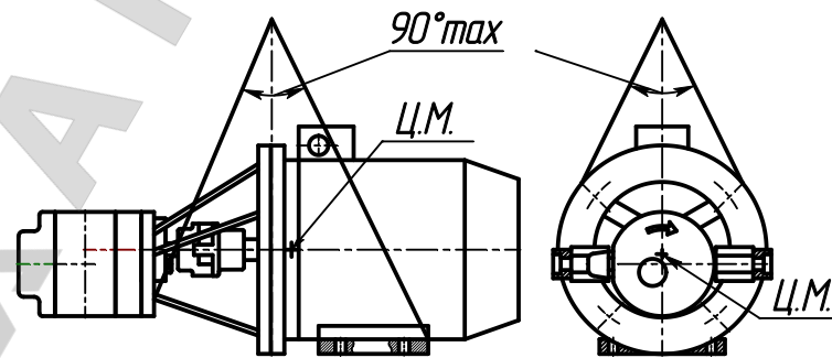
Схема строповки
