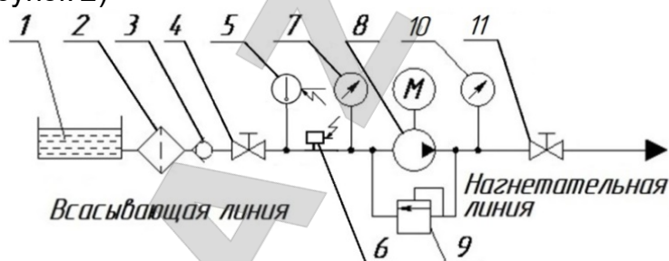
Рисунок 2 – Схема включения агрегата в сеть
