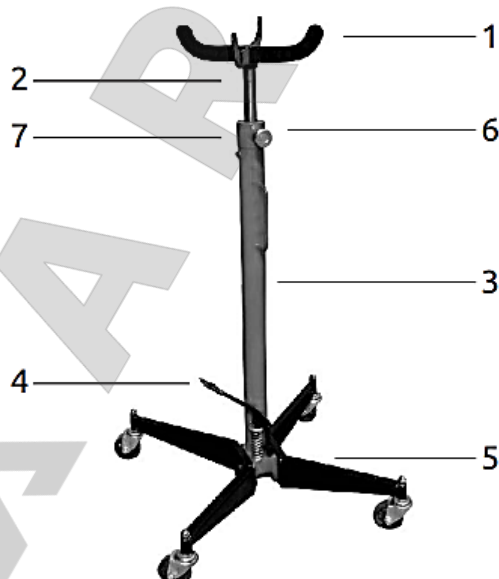
Устройство трансмиссионной стойки
