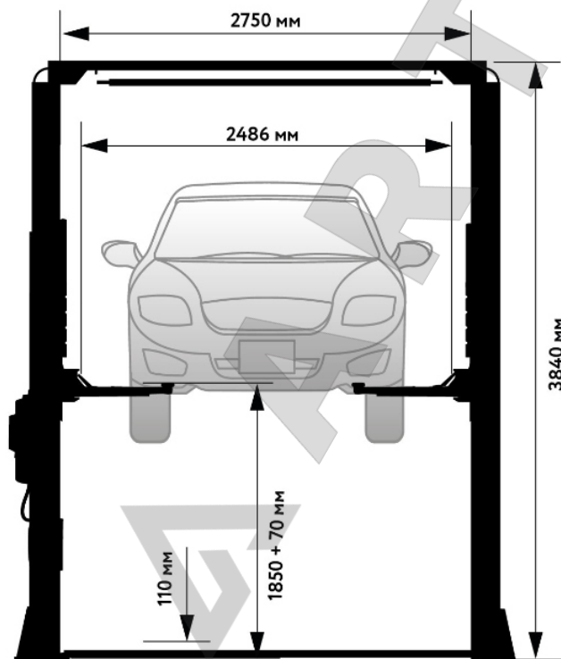
Чертеж WDK-529E
