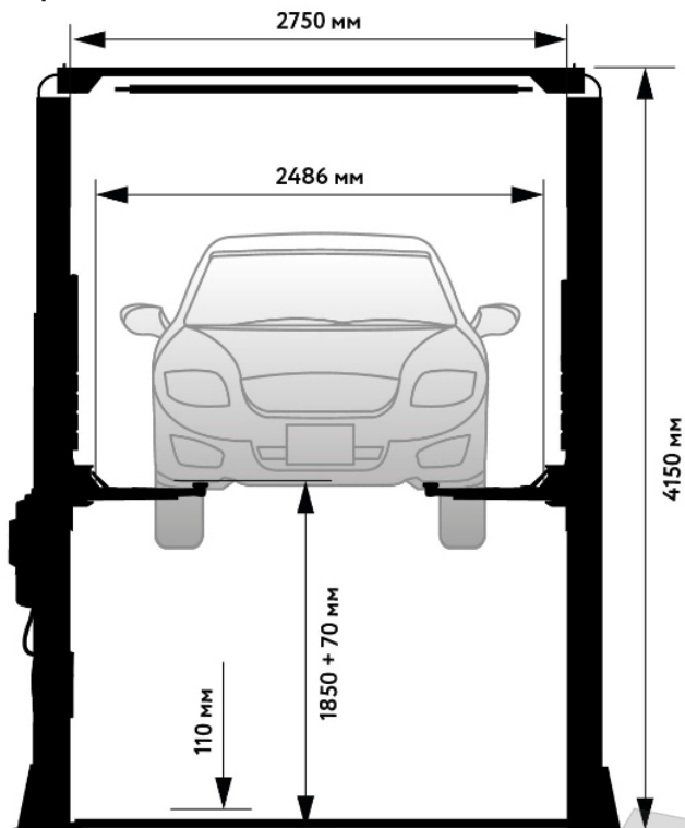
Чертеж WDK-529
