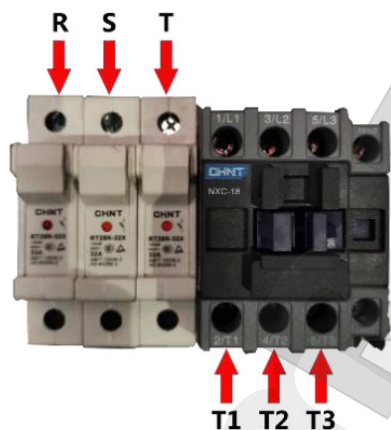
Терминал для подключения электропитания
