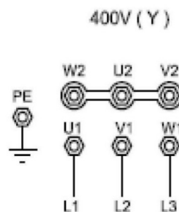
Подключение двигателя
