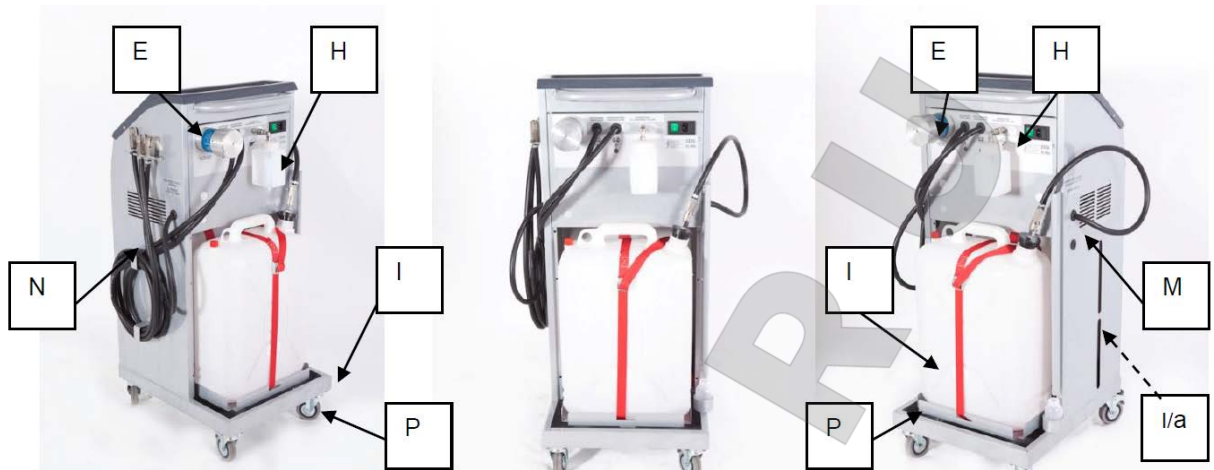
Рис. 5. Задняя сторона ATF4000.
