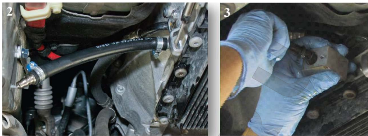
Рис. 21. Подсоединение станции к автомобилю (2) и (3).
