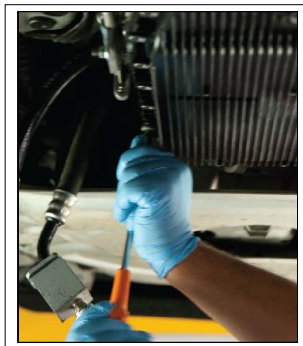
Рис. 22. Снятие масляного отстойника.
