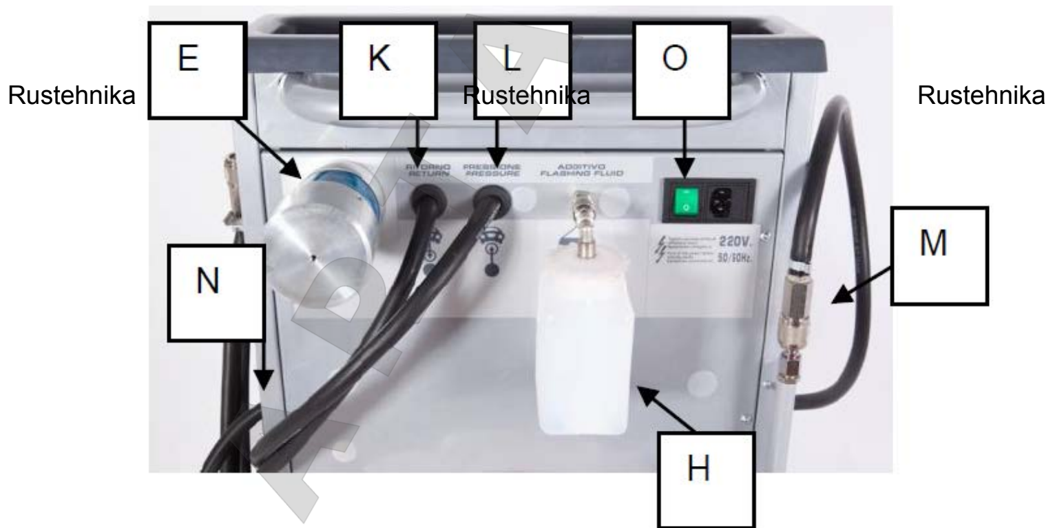
Рис. 6. Детализация задней панели ATF4000.
