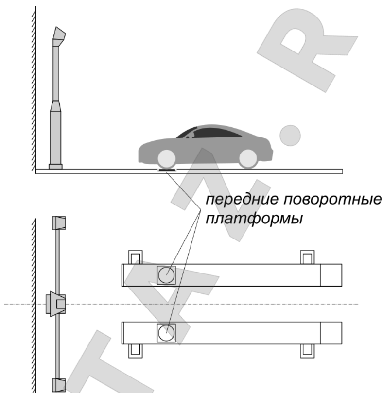
Рисунок Б.1 – Пример размещения прибора и автомобиля на рабочем месте
