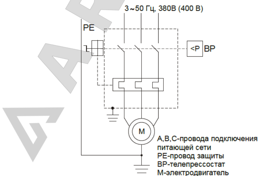
Рисунок 2 – Схема электрическая принципиальная
