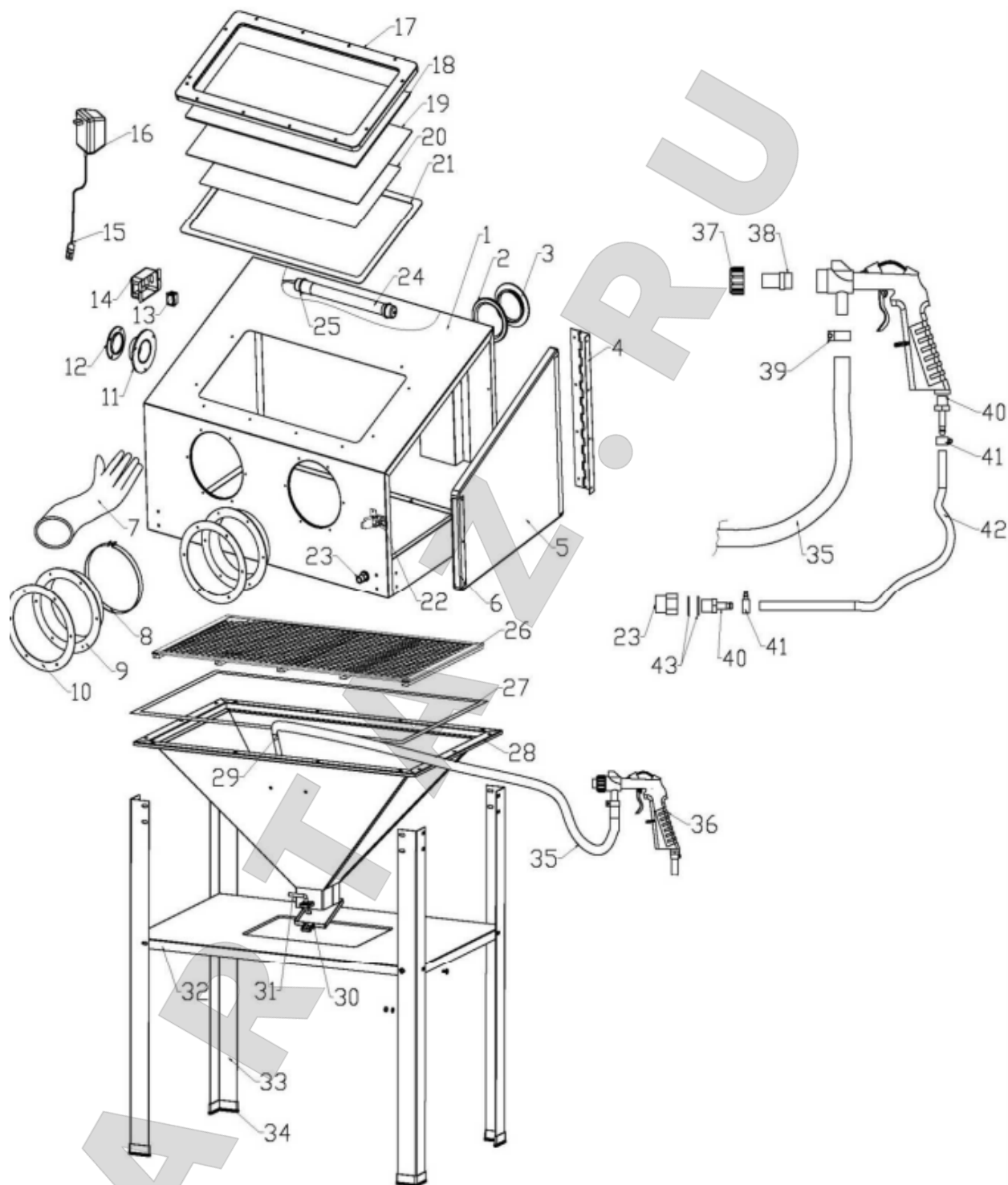
Рис. 3. Устройство изделия.
