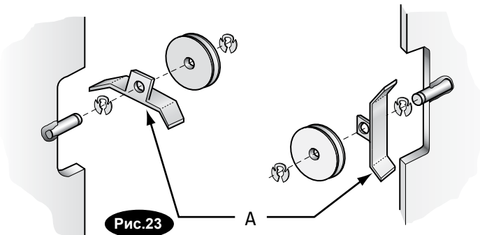
Рис. 23 - сборочные части A Крышки шкива
