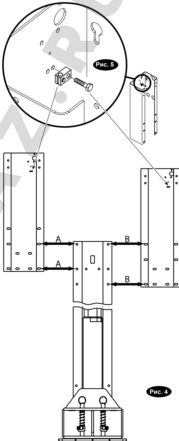
Рис. 4 - сборочные части
