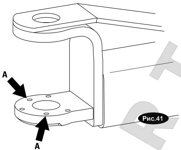
Рис. 41 - сборочные части
