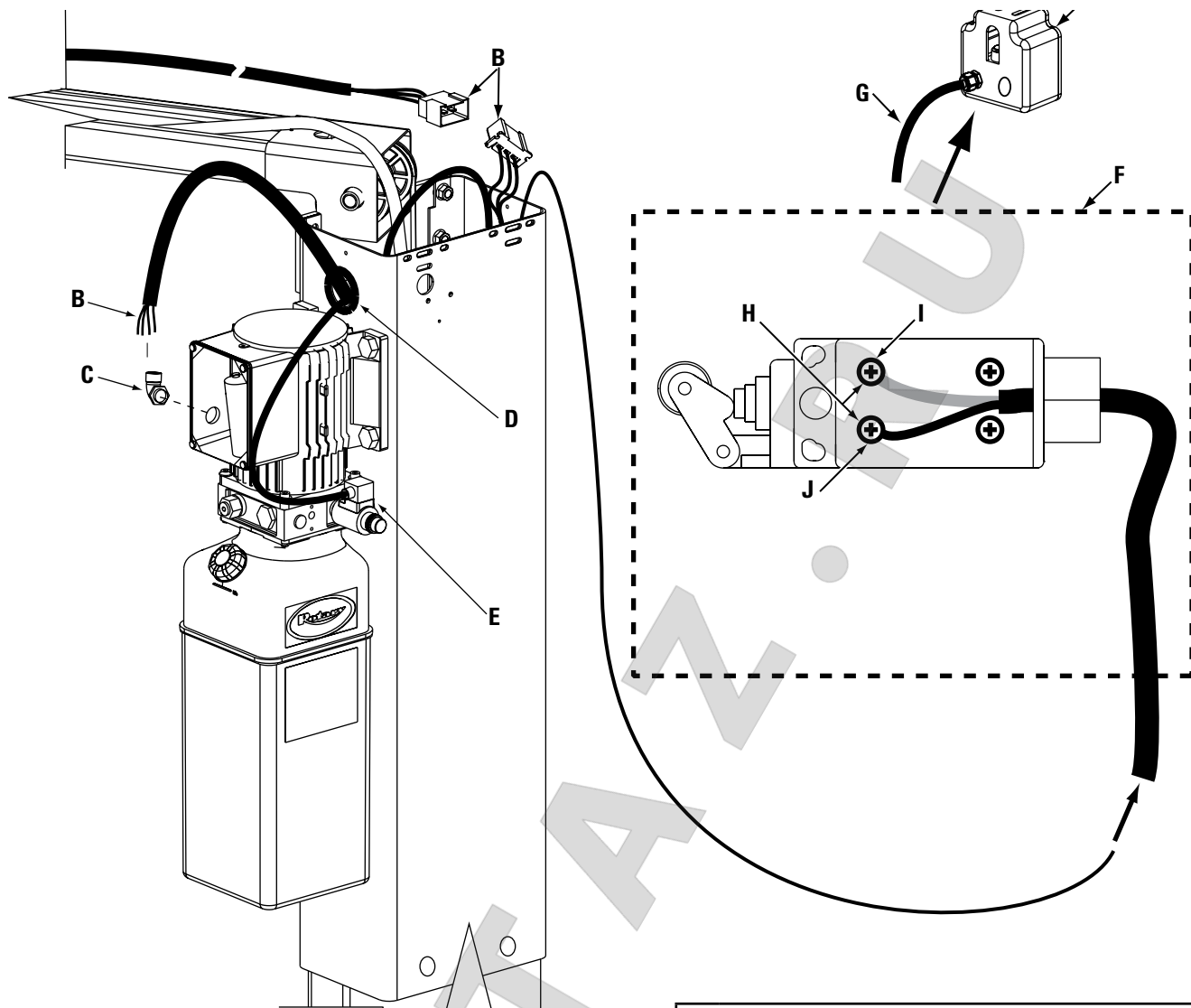
Рис. 34 - сборочные части
