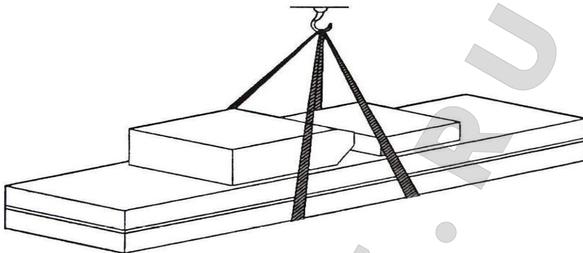
Рис. 1 Стрповка оборудования
