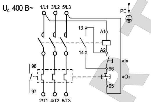
Схема электрическая контакторов с катушкой управления 400 В-
