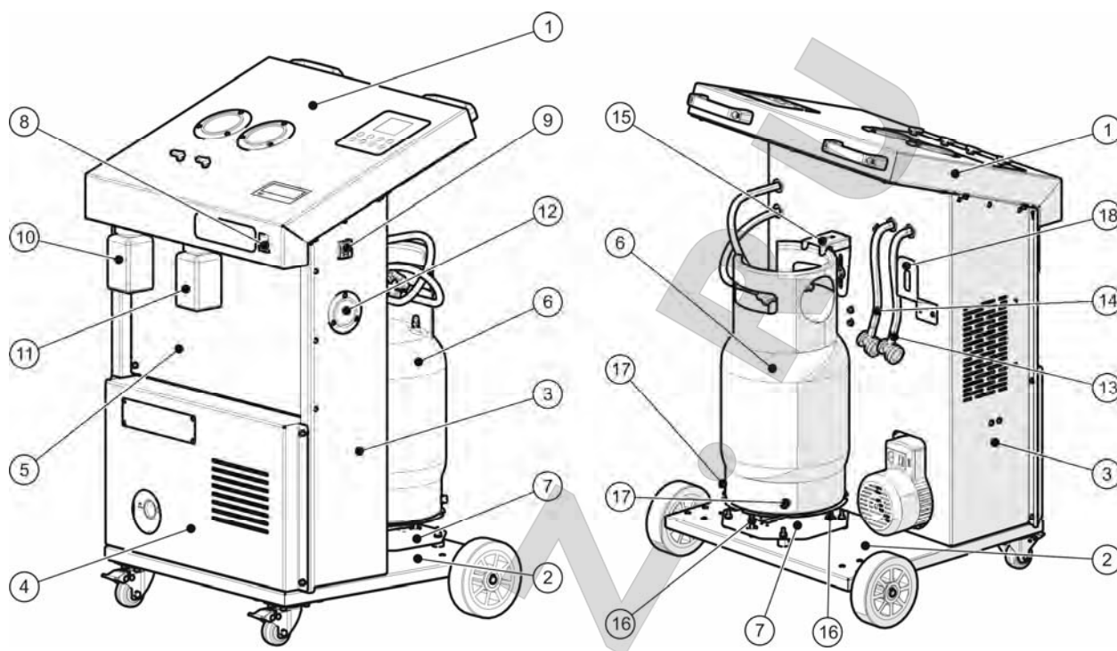
Рис. 2 Основные элементы станции ODA-360AP
