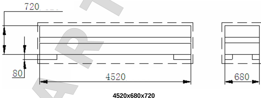
Габаритные размеры упаковки
