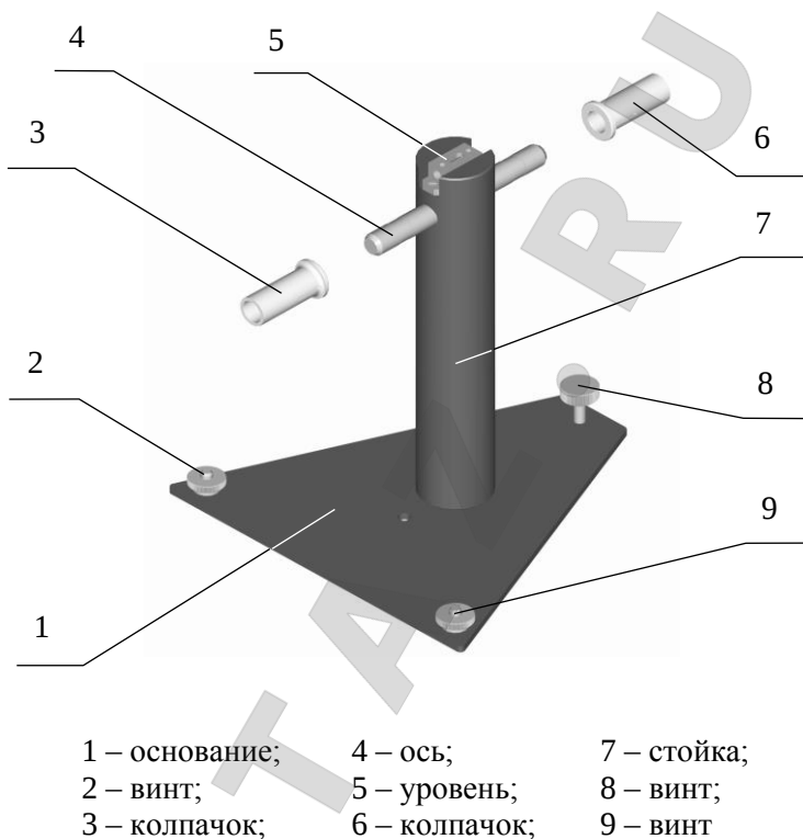
Рисунок 11 – Общий вид контрольной стойки
