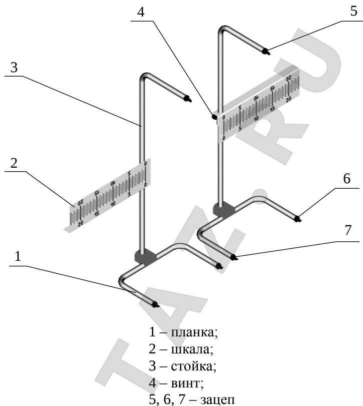
Рисунок 8 – Общий вид индикаторов
