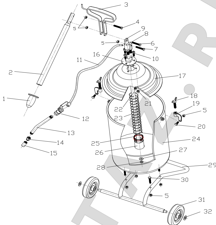
Чертеж – схема
