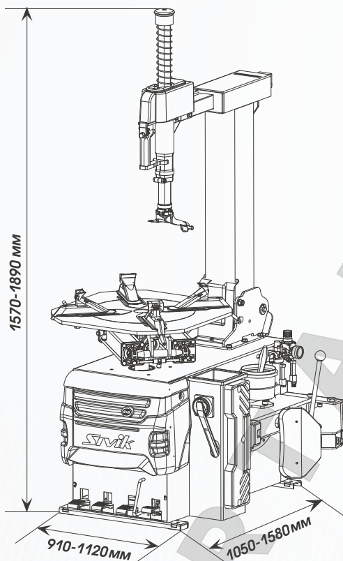
Рисунок 4 Установка стенда
