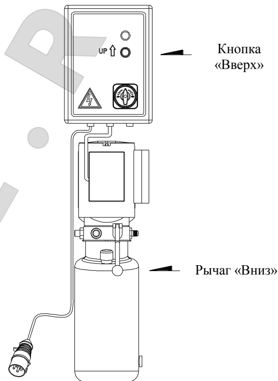
Рис. 32 Органы управления
