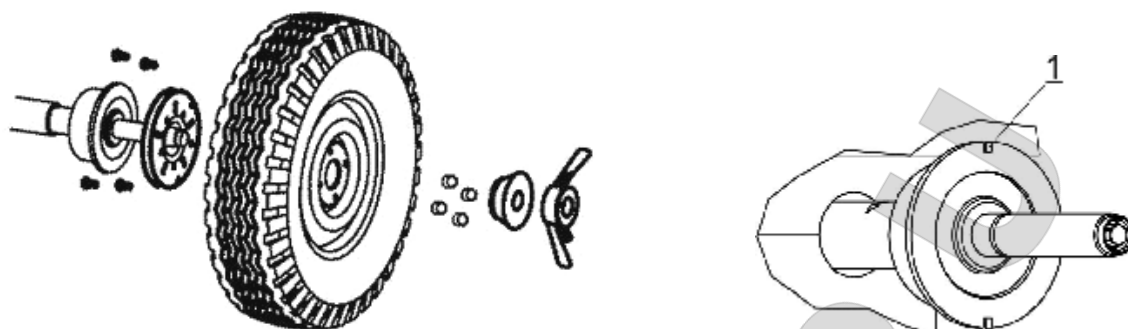
д – установка на адаптер фланцевый
