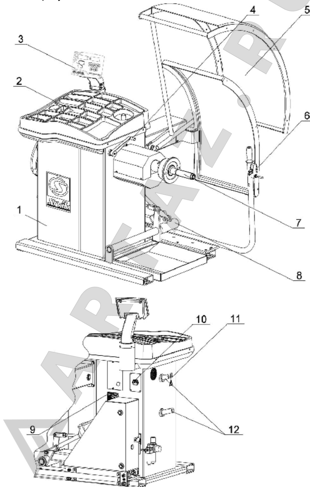
Рисунок 4.1 – Внешний вид станка
