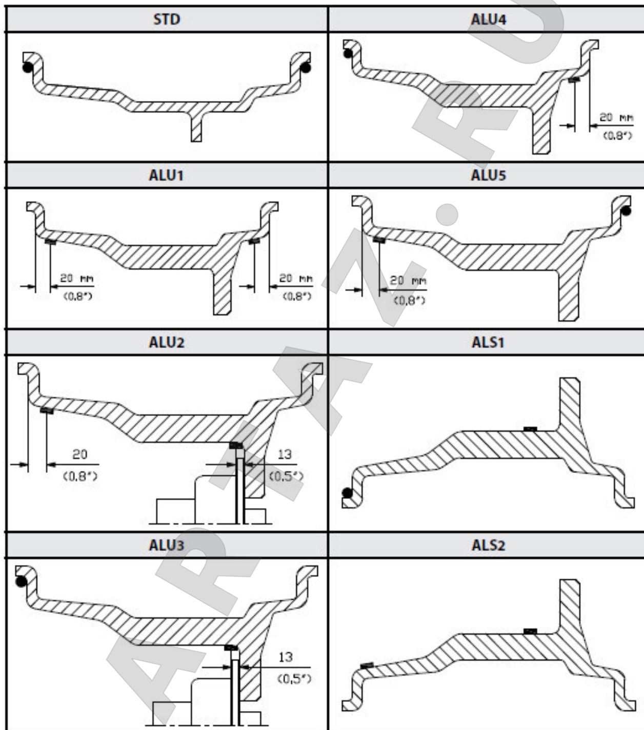
Рис. 3.1 Положение грузов в различных типах программ вдоль участка диска
