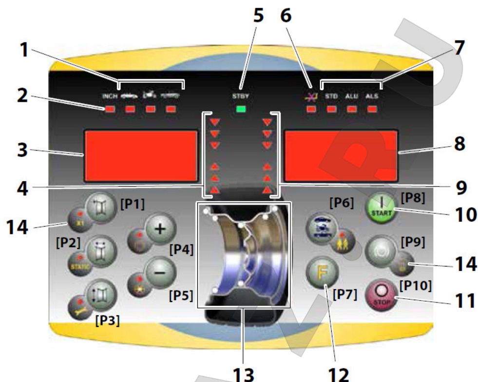
Рис. 1 Панель управления
