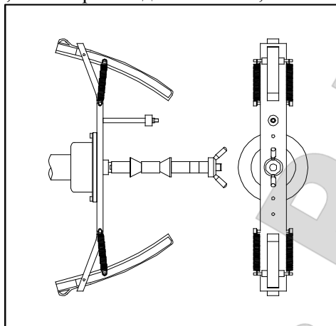
Рис. 4.3 Установка калибровочного грузика на внешней стороне адаптера для МOTO колес на валу (фаза Cal 3)
