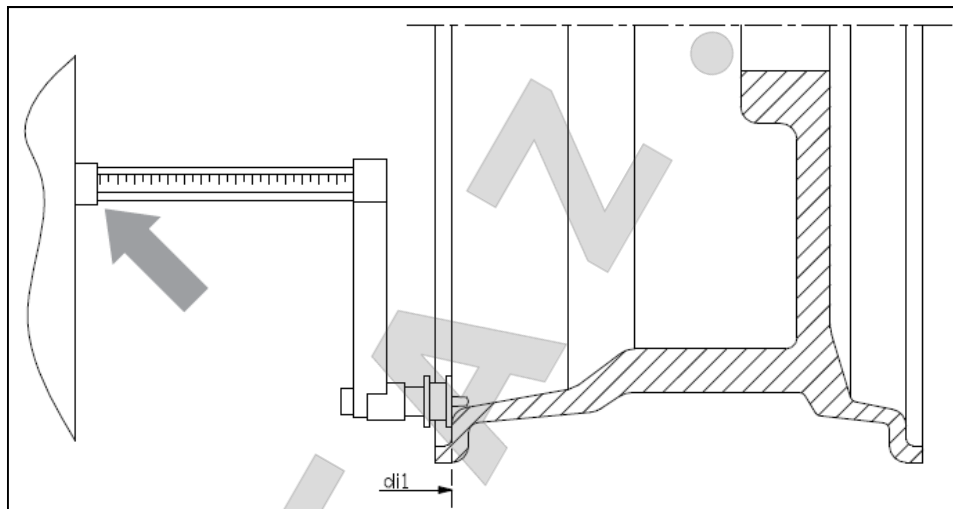
Рис. 3.4 Ручное измерение расстояния до колеса в программе ALS1
