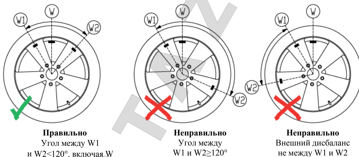
Рис. 6.1 Правильное и неправильное расположение скрытых грузиков
