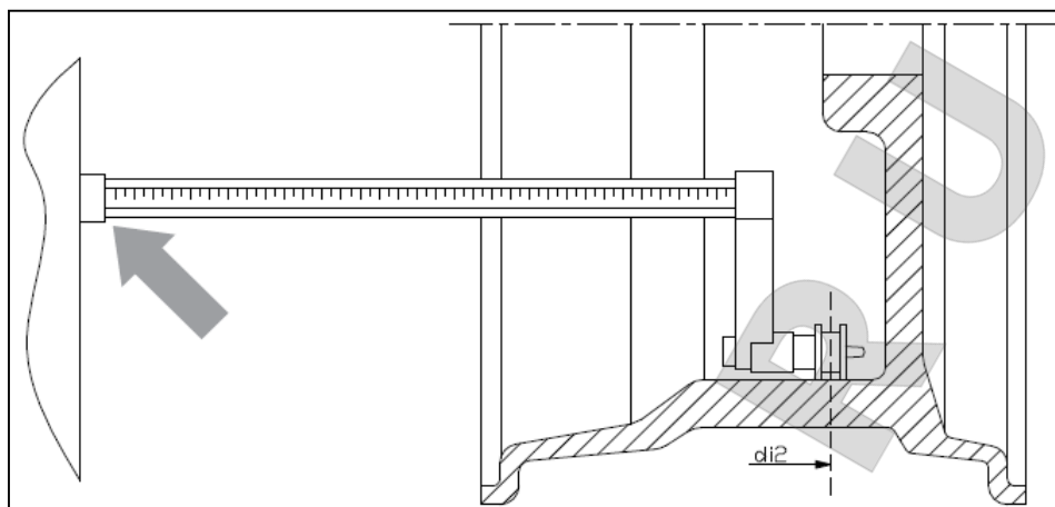
Рис 3.6 Ручное измерение расстояния до внешней плоскости в программах ALS1 и ALS2
