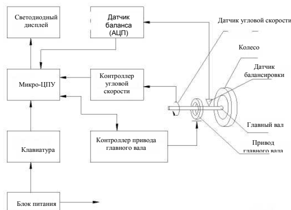
Рис. 3 Функциональная блок-схема балансирующего станка CB1930E
