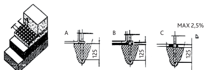
Рис. 3. Крепление рамы станка к полу анкерными болтами.
