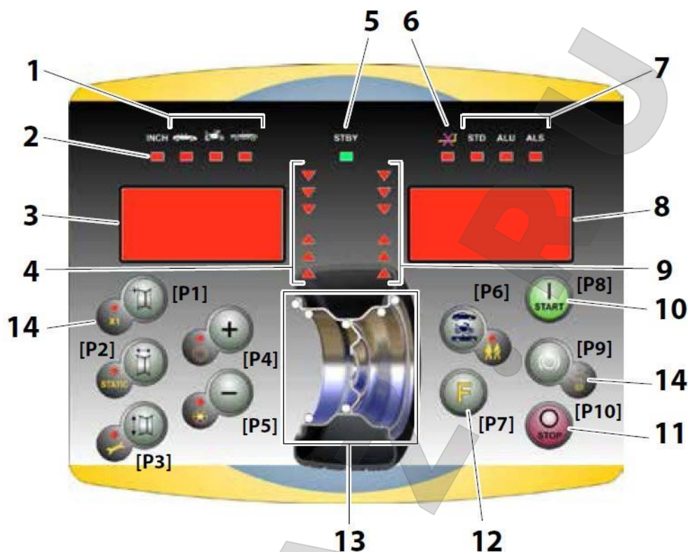
Рис. 1 Панель управления
