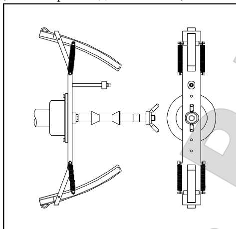
Рис. 4.3 Установка калибровочного грузика на внешней стороне адаптера для МОТО колес на валу (фаза Cal 3)
